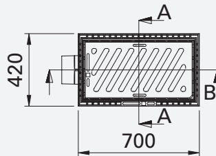
BOVENAANZICHT
