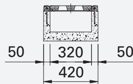
DOORSNEDE A-A
