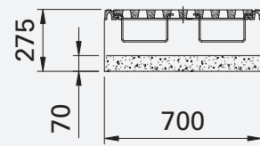
DOORSNEDE A-A TUSSENSTUK
