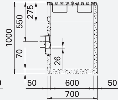
DOORSNEDE A-A ONDERBAK-EINDSTUK
