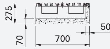
DOORSNEDE A-A BEGINSTUK
