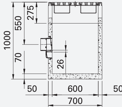
DOORSNEDE A-A ONDERBAK-TUSSENOPZETSTUK
